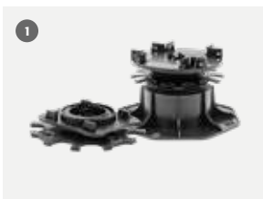
Terrassenlager MICRO & CLIP Höhenverstellbarkeit 10 - 225 mm, gleicht Gefälle des Untergrundes bis zu 8 % aus
